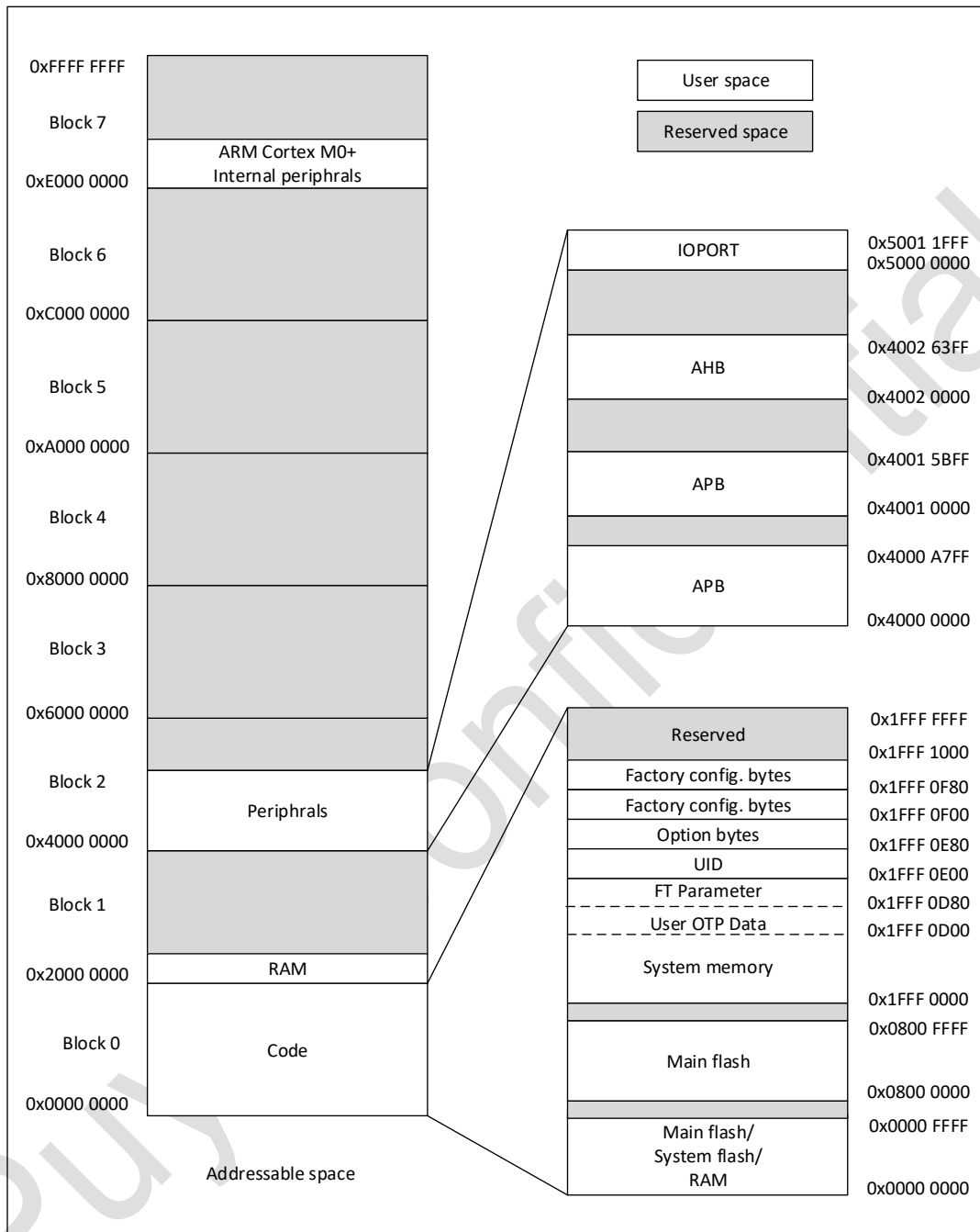
图 3-8 存储器映射
