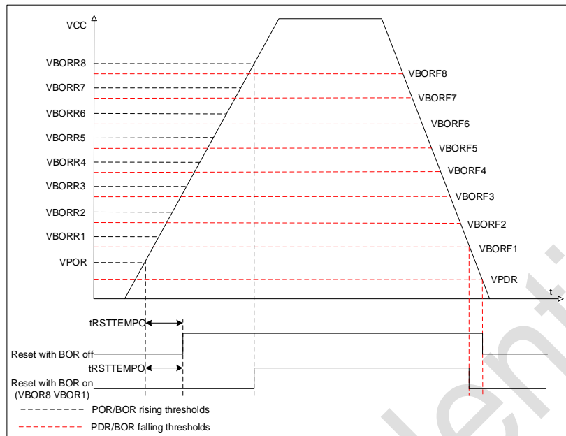
图 2-3 POR/PDR/BOR 阈值
