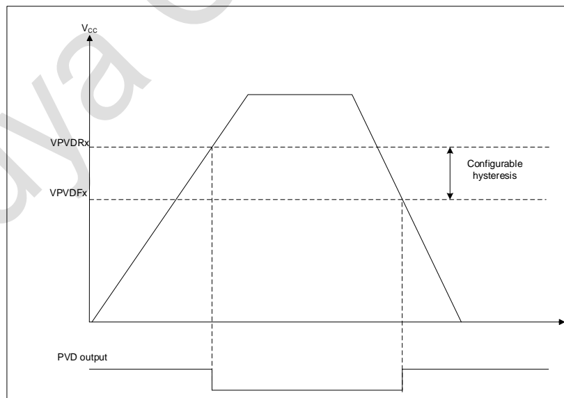
图 2-4 PVD 阈值
