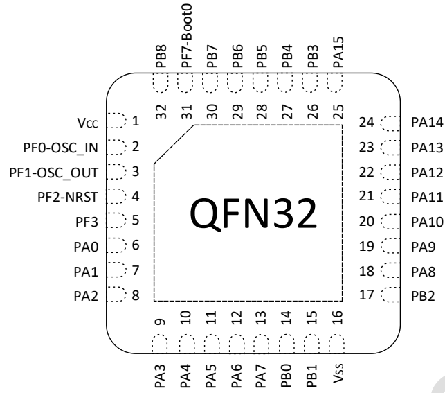
图 3-5 QFN32 Pinout1 PY32F031K1xU (Top view)
